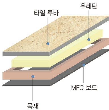
타일 패널 (칸막이) 구성도
