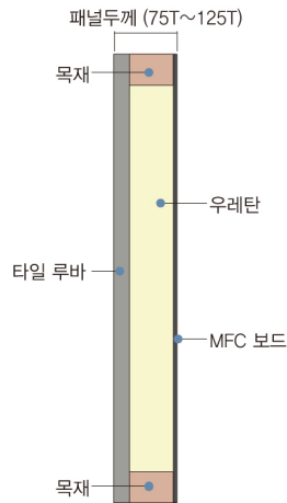
타일 패널 단면
